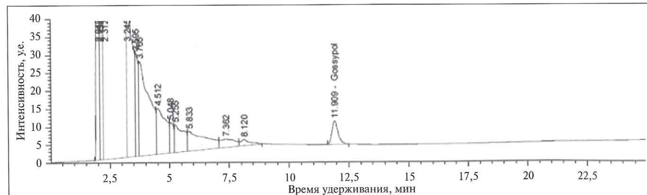
Рис. 3. Хроматограмма смеси госсипола с субстанцией после кислотного гидролиза
