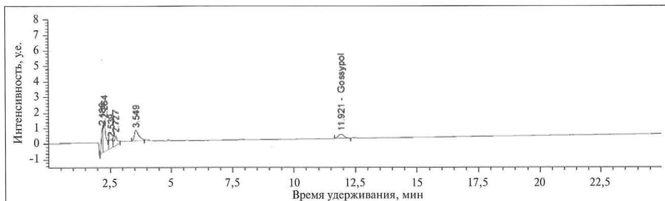
Рис. 4. Хроматограмма раствора госсипола в концентрации, соответствующей пределу количественного определения
