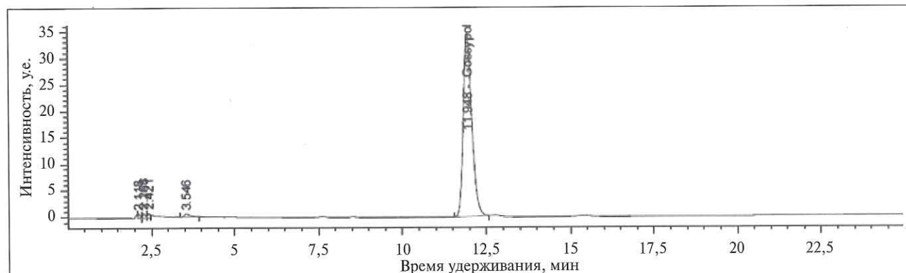
Рис. 2. Хроматограмма раствора сравнения (стандартный образец госсипола)
