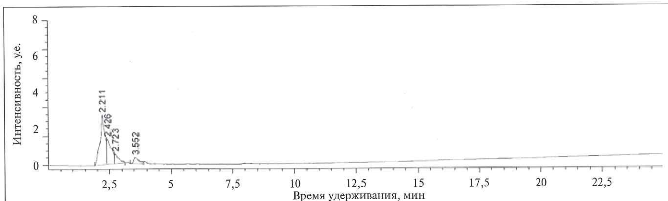
Рис. 1. Хроматограмма подвижной фазы (бланк)
